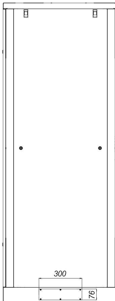
Вид слева
